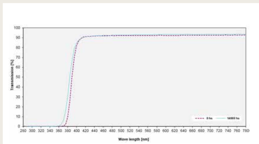
Abb. 1: Transmissions-Spektrum von PLEXIGLAS® Folie 0F011 vor und nach künstlicher Bewitterung nach DIN EN ISO 4892-2, Methode A, Zyklus 1
