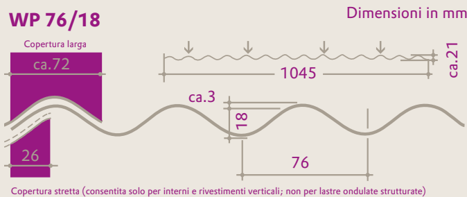
Sezione trasversale di PLEXIGLAS® Heatstop Cool Blue WP 76/18 (dimensioni in mm)
