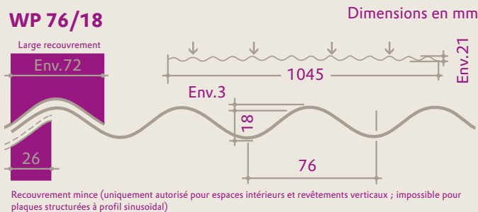
Coupe transversale d'une plaque PLEXIGLAS® Heatstop Opal WP 76/18 (dimensions en mm)
