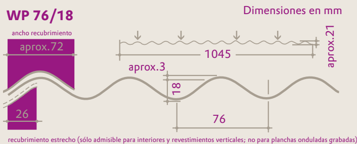
Sección de la plancha ondulada PLEXIGLAS® Heatstop Ópalo WP 76/18 (dimensiones en mm)
