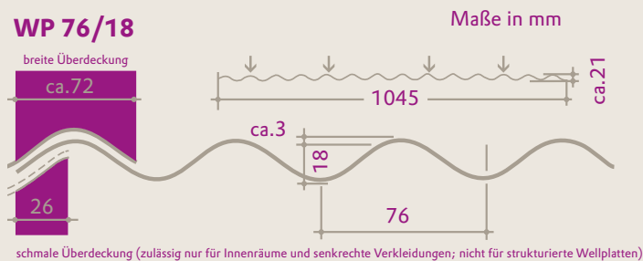
Querschnitt der PLEXIGLAS® Heatstop Opal WP 76/18 (Maße in mm)
