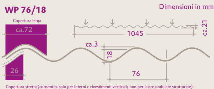
Sezione trasversale di PLEXIGLAS® Resist WP 76/18 (dimensioni in mm)
