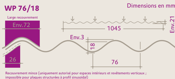
Coupe transversale d'une plaque PLEXIGLAS® Resist WP 76/18 (dimensions en mm)
