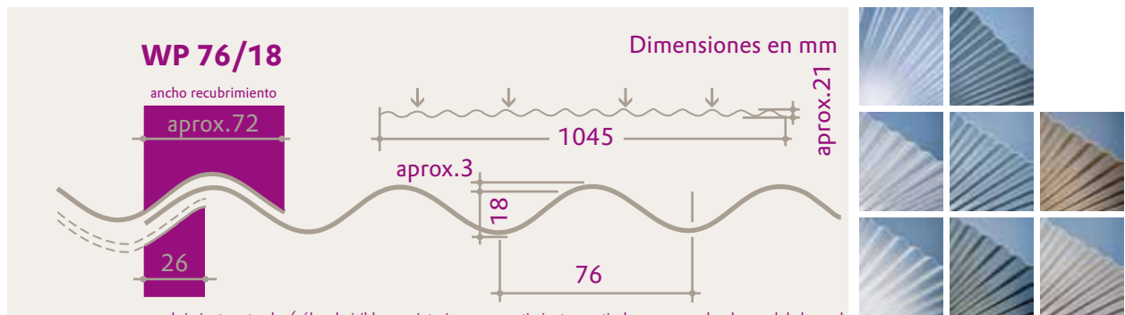
Sección de la plancha ondulada PLEXIGLAS RESIST® WP 76/18 (dimensiones en mm)
