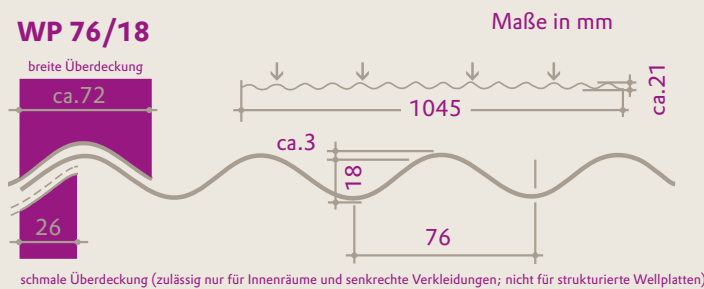
Querschnitt der PLEXIGLAS® Resist WP 76/18 (Maße in mm)
