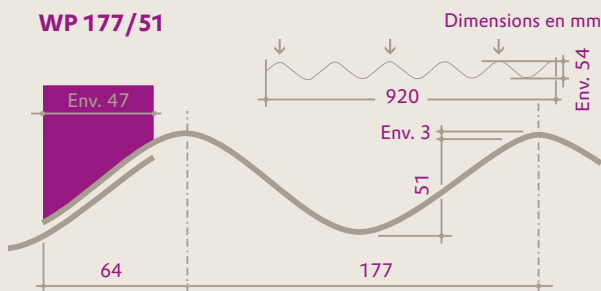
Coupe transversale d'une plaque PLEXIGLAS® Resist WP 177/51 (dimensions en mm)
